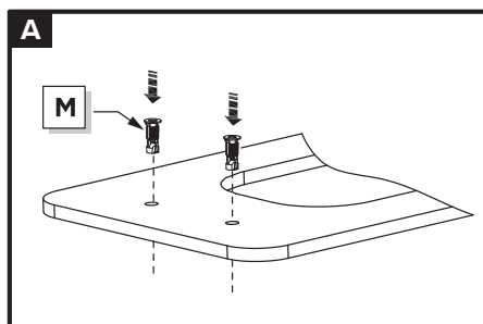
Sett inn de ekspanderende gummiboltene i hullene i veggskålen
